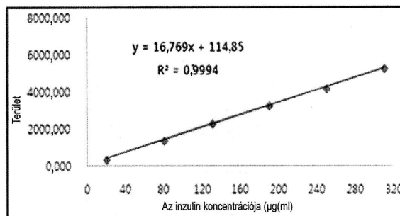
Az inzulin standard kalibrációs görbéje
